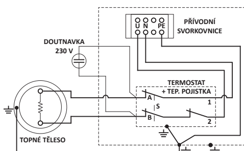
Zapojení 1x230 V~ tělesa 1-1,5 kW s jednofázovým termostatem
