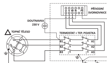
Zapojení do trojúhelníku 3x400 V~ tělesa 6-12 kW s trojfázovým termostatem
