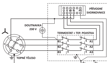
Zapojení do hvězdy 3x230 V~ tělesa 2-6 kW s trojfázovým termostatem
