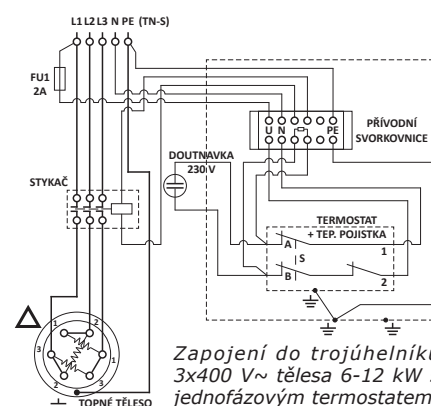
Zapojení do hvězdy 3x230 V~ tělesa 2-6 kW s jednofázovým termostatem
