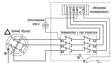
Zapojení do trojúhelníku 3x400 V~ tělesa 7,5-12 kW s trojfázovým termostatem
