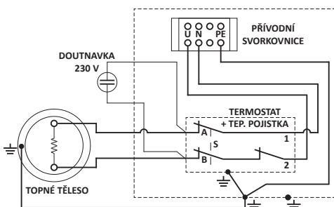
Zapojení 1x230 V~ tělesa 2,4-3 kW s jednofázovým termostatem
