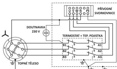
Zapojení do hvězdy 3x230 V~ tělesa 2,4-6 kW s trojfázovým termostatem
