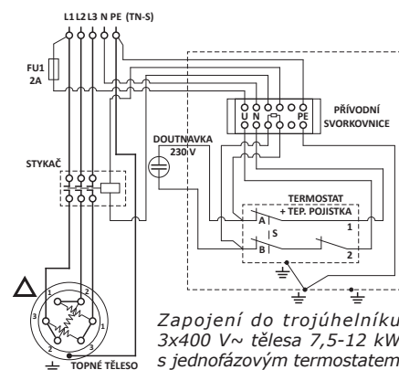
Zapojení do hvězdy 3x230 V~ tělesa 2,4-6 kW s jednofázovým termostatem
