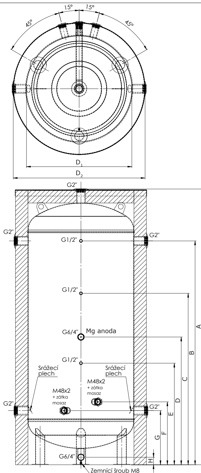
Obr. 3 AZN VS 750 - 1 000 S s izolací
