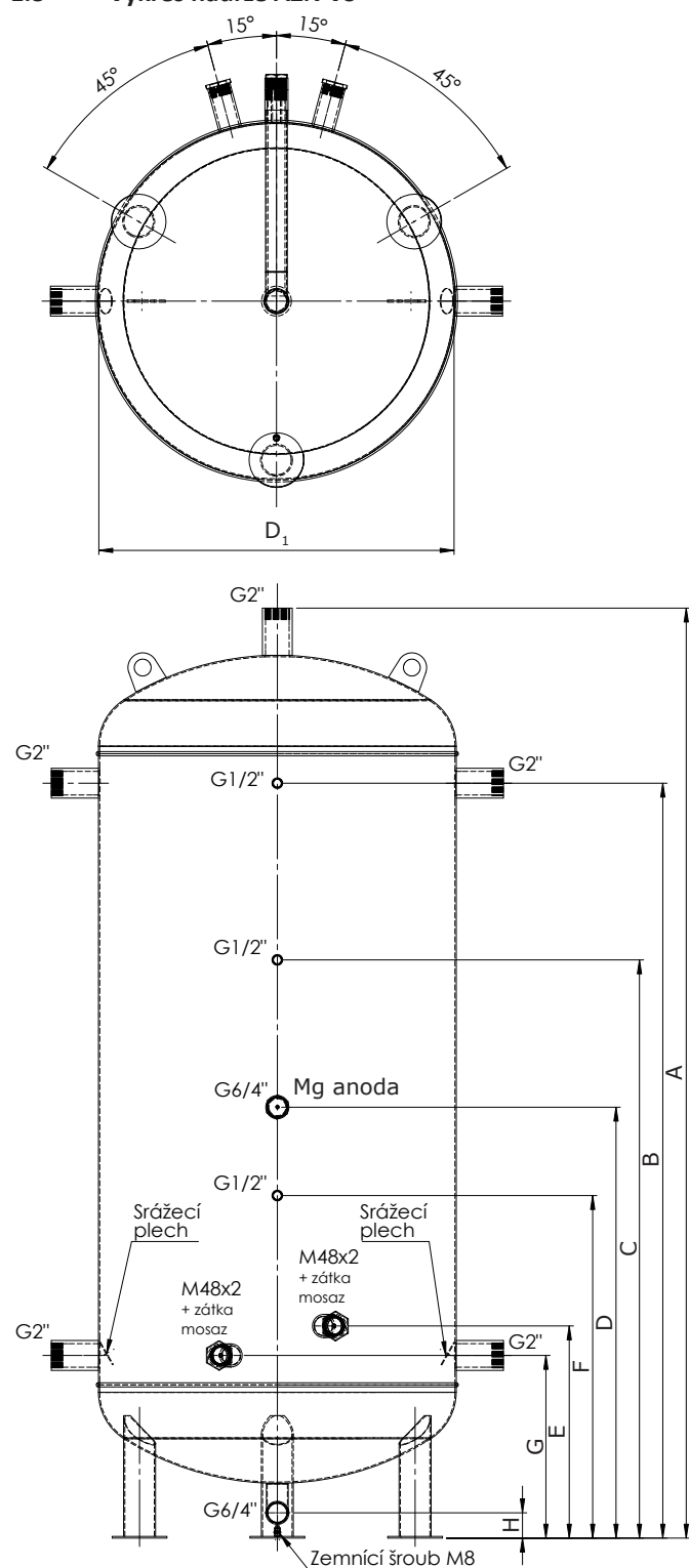
Obr. 2 AZN VS 750 - 1 000 S bez izolace
